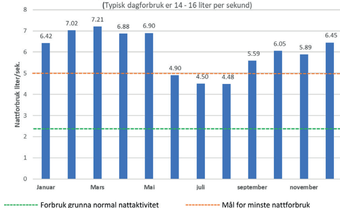
Utvikling nattforbruk/lekkasjar målt frå Lyshol 2021 (Typisk dagforbruk er 14 - 16 liter per sekund)
